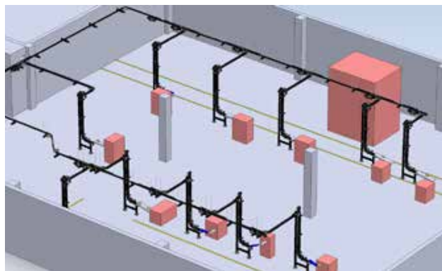
Slika 1 : Transportni sistemi Dorner v Herbariumu
