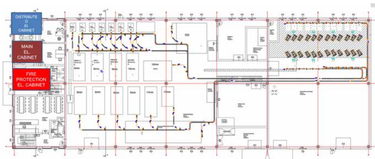
Slika 3 : Integracija sistemov za informatizacijo in digitalizacijo proizvodnje
